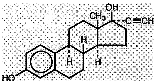
ETHINYL ESTRADIOL
